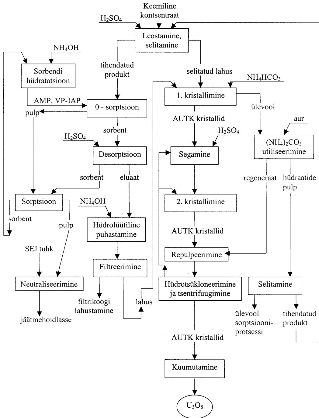
Joonis 6. Keemilise kontsentraadi hape-sorptsioon-töötlemise tehnoloogiline skeem
